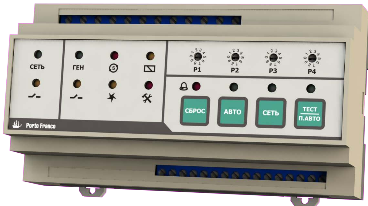
Рис. 5.1. Внешний вид контроллера АВР-КД
